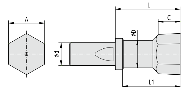
Sezione esagonale standard (E) Standard hexagonal section (E)
