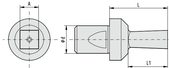
Sezione quadra standard (Q) Standard square section (Q)
