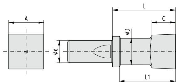
Sezione quadra standard (Q) Standard square section (Q)
