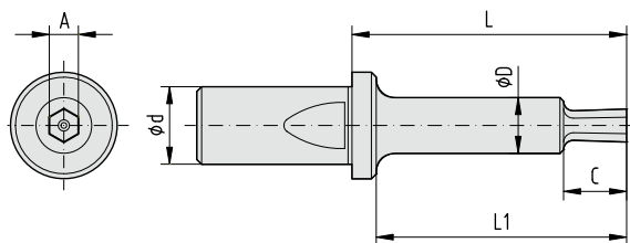
Sezione esagonale standard (E) Standard hexagonal section (E)
